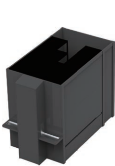
120ボックス仕様 FCNN1P-Z□□□ FCNF1P-Z□□□ 1400W×2440D×2100H
