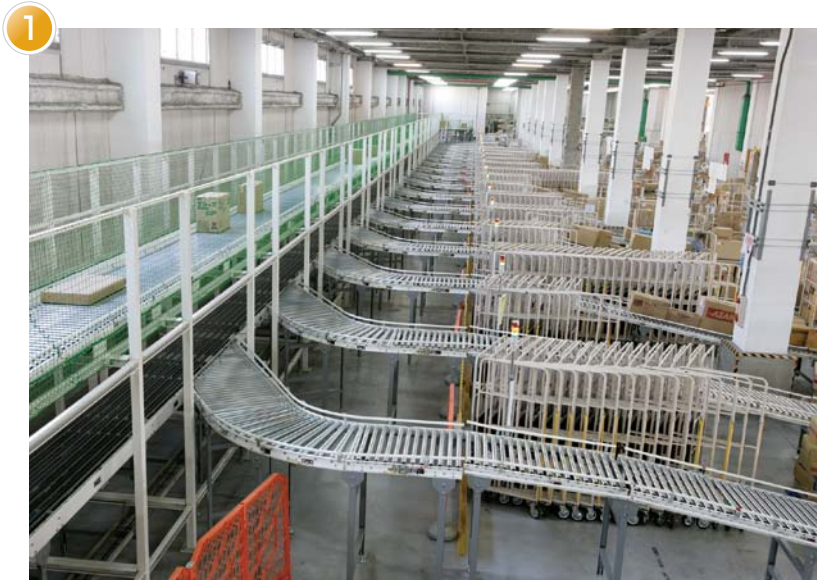
1 上段:シュート満載時の通過リターン用バイパスライン
